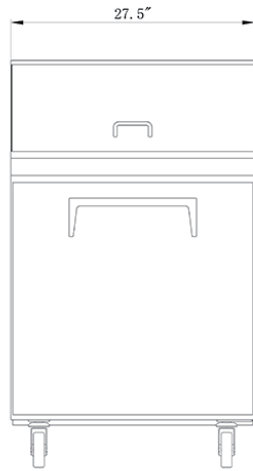
ELEVATION
