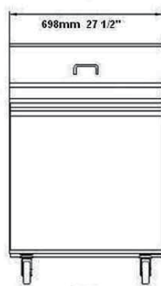
Elevation
