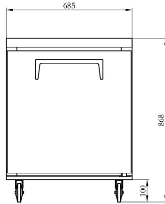
ELEVATION
