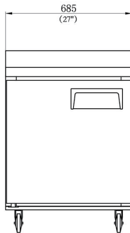
ELEVATION
