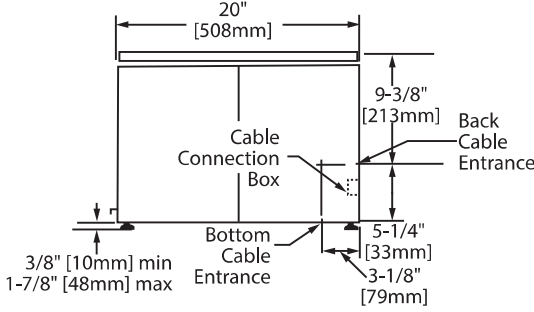
Counter Model E20-SPC
